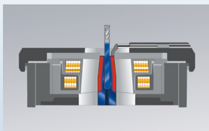
Petit outil/Utensile di piccole dimensioni
