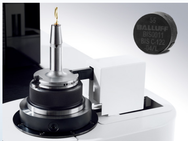
Après avoir mesuré l'outil, les données sont écrites sur le support de données Balluff (puce)/Dopo aver misurato l'utensile, i dati vengono trasferiti al supporto dati Balluff
