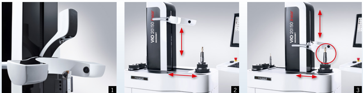
1: 2ème caméra pour régler le centre de rotation (optionnel)/Seconda telecamera per l'impostazione del centro di rotazione (opzionale) 2 + 3: Mouvement d'axe automatique par technologie linéaire très moderne/Assi con movimentazione completamente automatizzata secondo la più moderna tecnologia lineare
