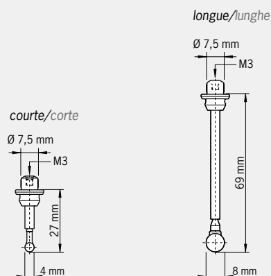
Touche de palpé/Astine tastatore
