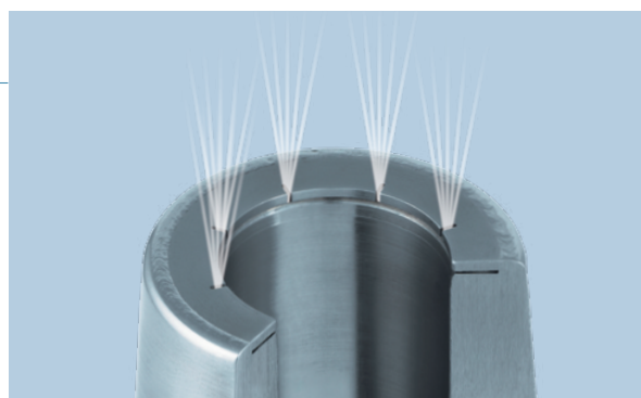
Perçage de conduits d’arrosage optimisé avec sortie du liquide par des fentes Système Cool Flash de HAIMER Fori per il passaggio del liquido refrigerante ottimizzati. Fuoriuscita del liquido attraverso le fessure Sistema Cool Flash di HAIMER
